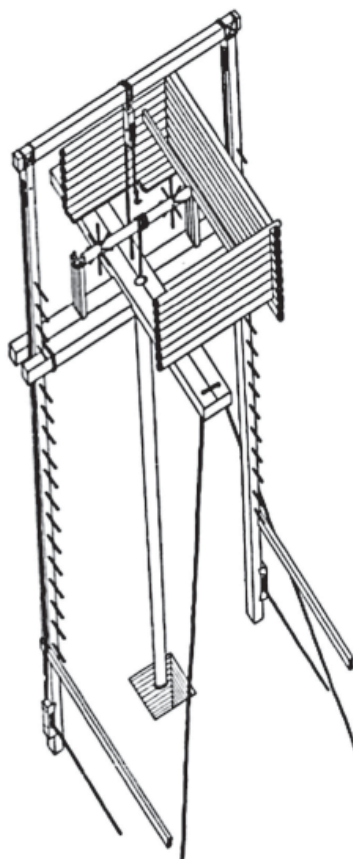
Чертеж буровой вышки по трактату XVI века
