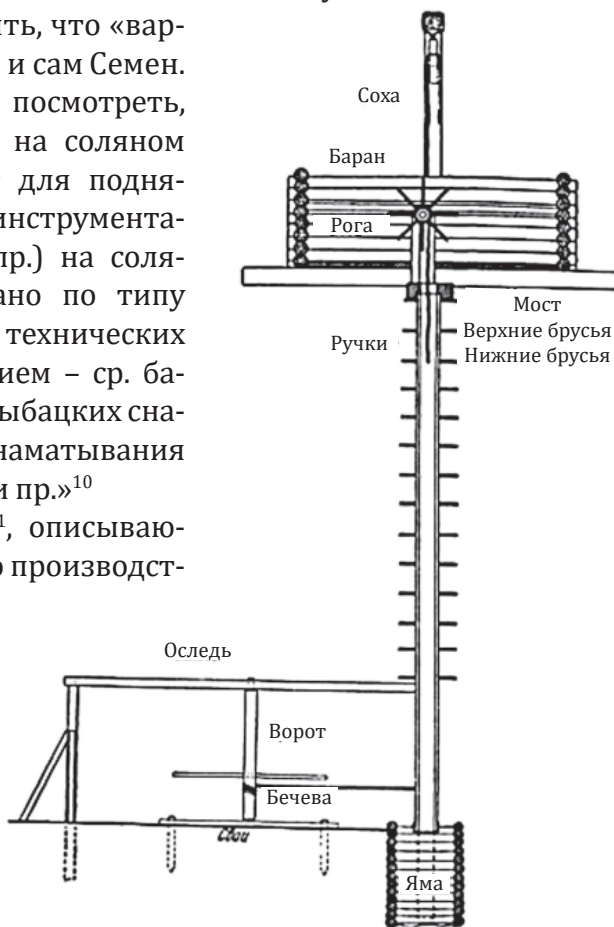
Баран на рисунке буровой соляной вышки
